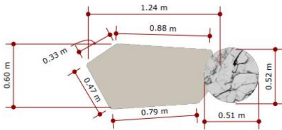
Vista Superior escala 1:20
